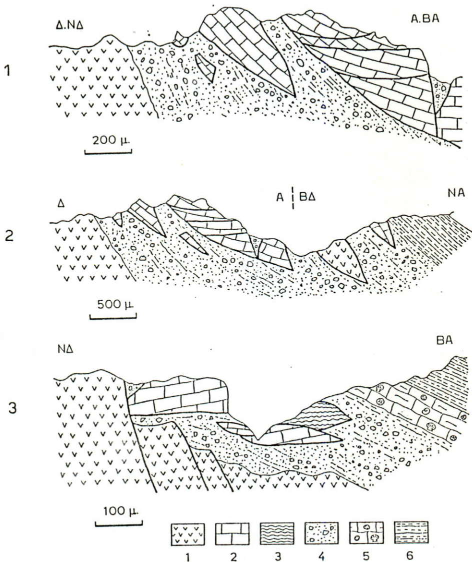
Σχ. 6. Σχηματικές γεωλογικές τομές στην περιοχή του Ορλιακά (1,2) και στην περιοχή Καταφυγίου (3), που δείχνουν τα τεκτονοϊζηματογενή φαινόμενα στη βάση της μόλασσας Επταχωρίου.
