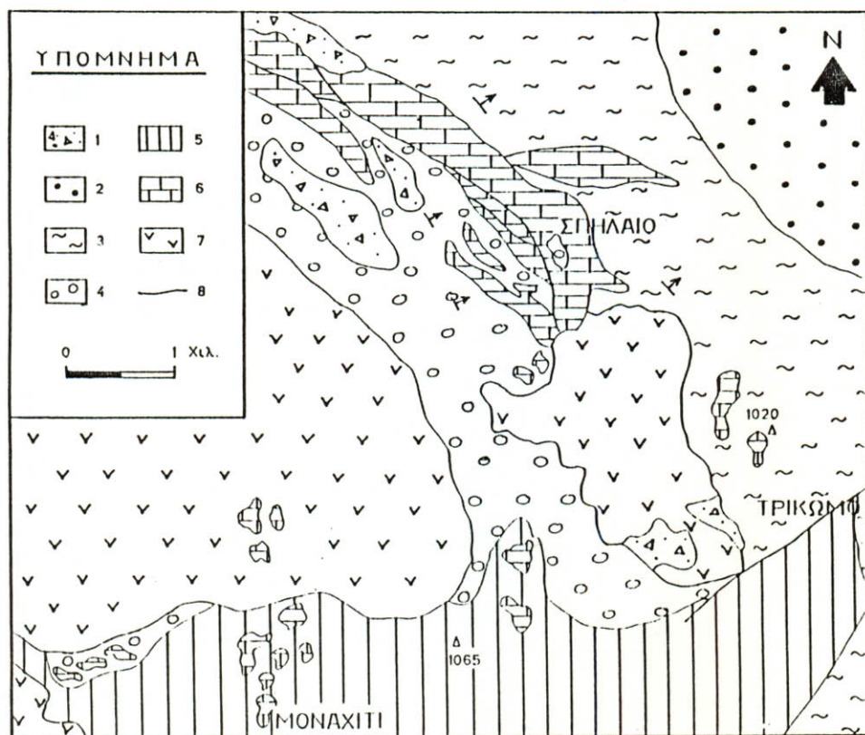
Σχ. 4. Αιλοποιημένος γεωλογικός χάρτης της περιοχής του Όρλιακα (βασιμμένος και στα στοιχεία του γεωλογικού χάρτη του Κουμαντάκη, 1980).
