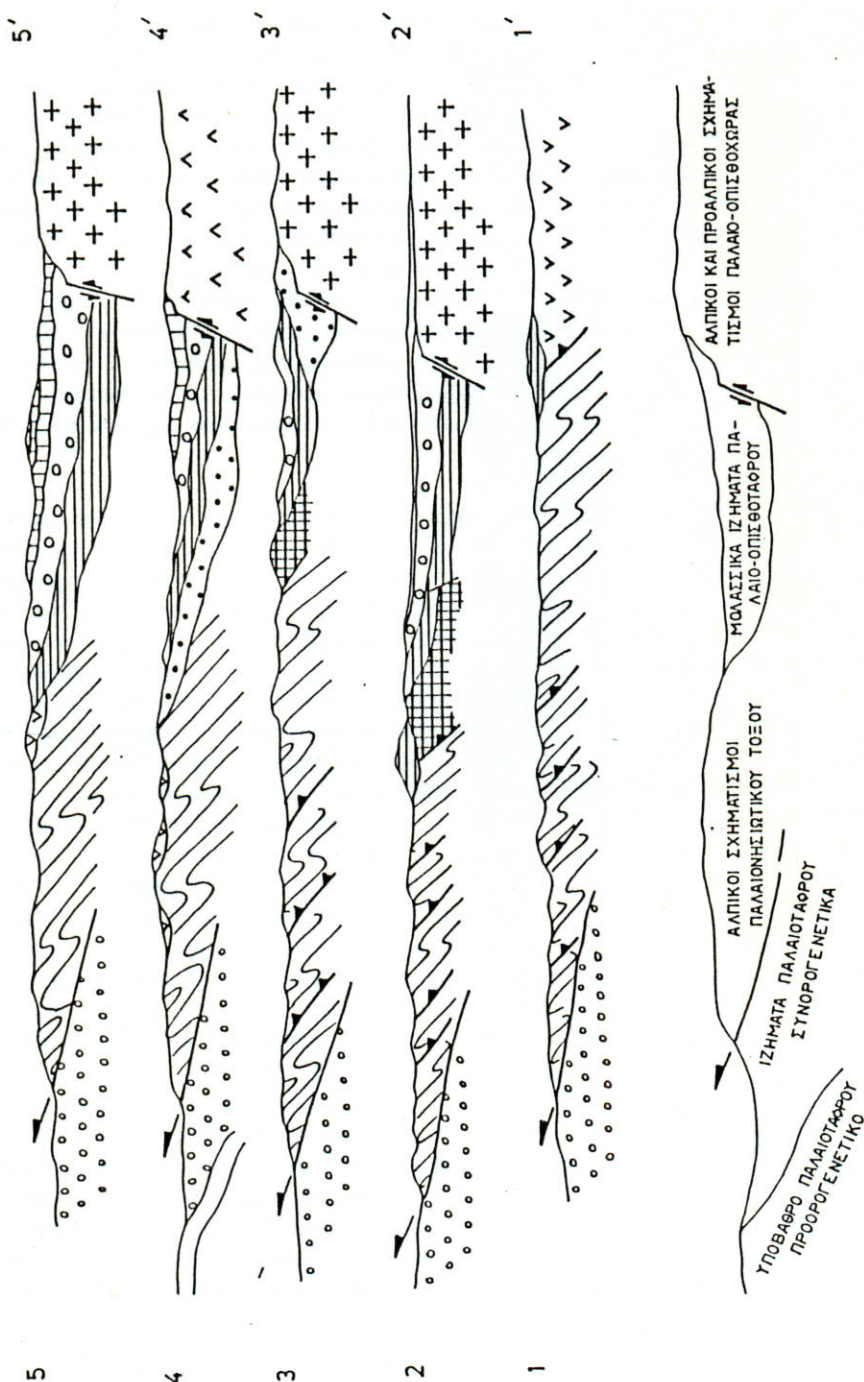
Σχ. 2. Πέντε εγκάρσιες τομές κατά μήκος της Μεσοελληνικής αλυσάκας και της οροσειράς της Πίνδου που δείχνουν τη συνολική δομή (οι θέσεις των τομών σημειώνονται στο χάρτη του Σχ. 1) και μία γενικευμένη σχηματική με βάση την παλαιογεωδυναμική ερμηνεία.
