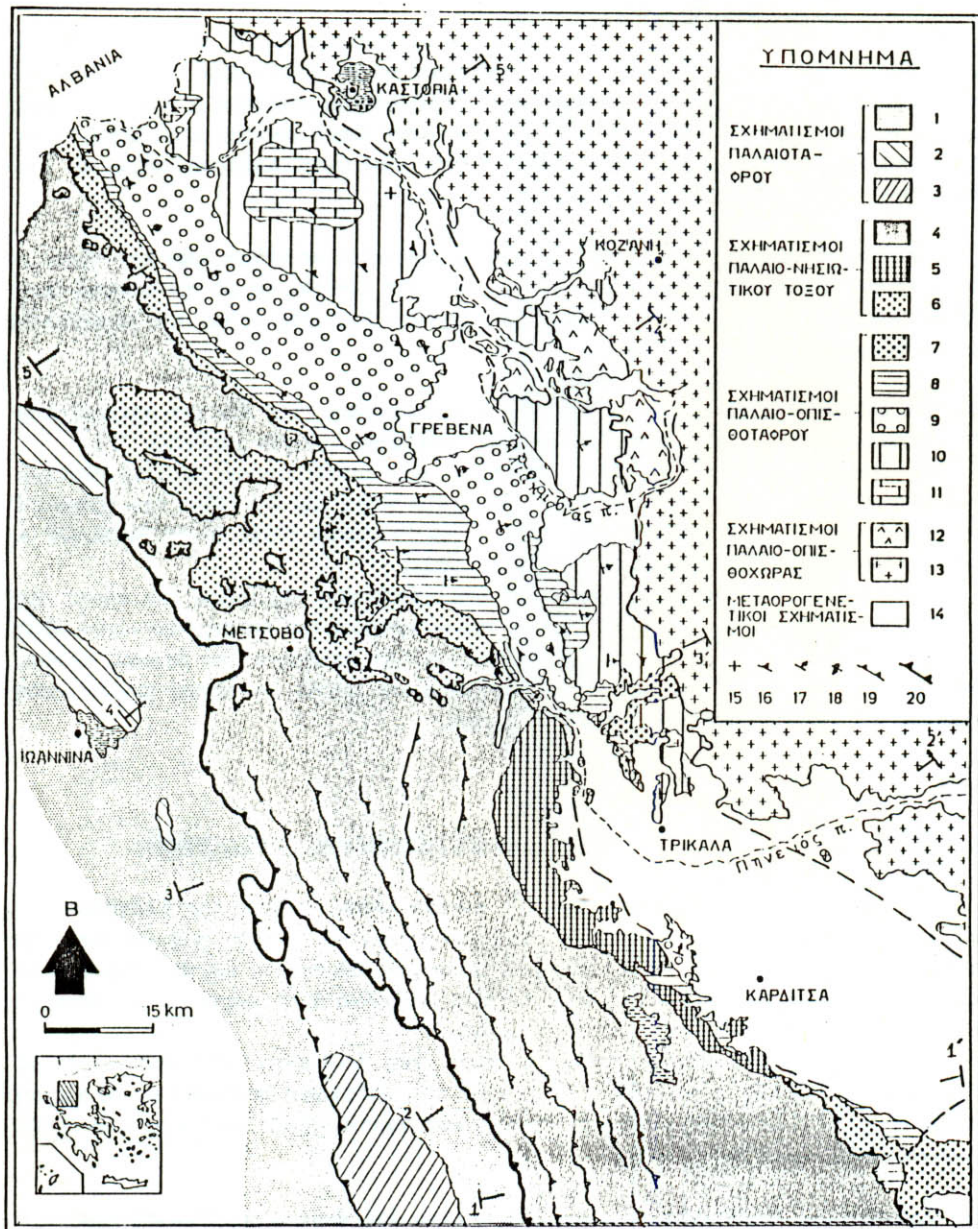
Σχ. 1. Απλοποιημένος γεωλογικός χάρτης της Μεσσελληνικής Αύλακας και των γειτονικών της περιοχών με ταξινόμηση τους σύμφωνα με την παλαιογεωδυναμική τους θέση στα πλαίσια του εξελισσόμενου ορογενετικού τόξου των Ελληνίδων. 1. Ενιαίος φλύσχης Γαβρόβου-ονου 2. Ανθρακικοί σχηματισμοί Ιονίου 3. Ανθρακικοί σχηματισμοί Γαβρόβου 4. Σχηματισμοί Πίνδου 5. Ενότητα Δυτικής Θεσσαλίας 6. Οφιόλιθοι Βορ. Πίνδου, Οφιόλιθοι Όρθρου 7. Σχηματισμός Κρανιάς 8. Σχηματισμός Επιταχωρίου 9. Σχηματισμός Πενταλόφου 10. Σχηματισμός Τσοτυλίου 11. Σχηματισμός Όντρια 12. Οφιόλιθοι Βούρινου 13. Κρυσταλλικό υπόβαθρο Πελαγονικής s.l. 14. Πλειο-τεταρτογενές 15. Οριζόντια στρώματα 16. Κλίση στρωμάτων ως 15° 17. Κλίση στρωμάτων μεγαλύτερη από 15° 18. Ανάστροφα στρώματα. 19. Εφριπτεύσεις, 20. Επωθήσεις.
