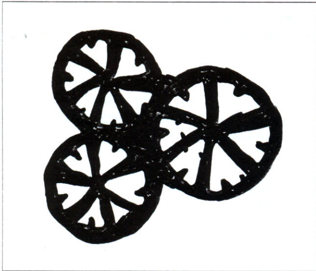
Figure 4 - Astrocoenia palmata (CATULLO). Schéma de l'arrangement des septes. Astrocoenia palmata (CATULLO). Septal arrangement.
