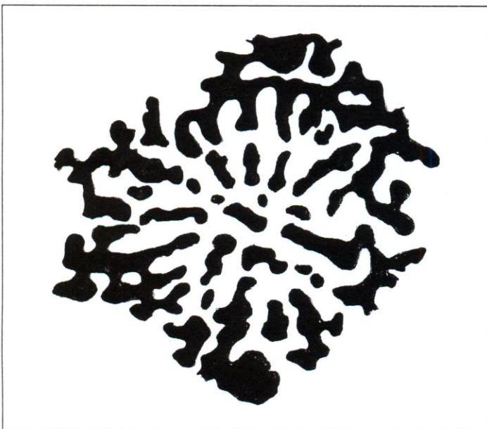
Figure 6 - Porites minuta REUSS. Schéma de l'arrangement des septes. a : colu- melle. Porites minuta REUSS. Septal arran- gement. a : columella.
