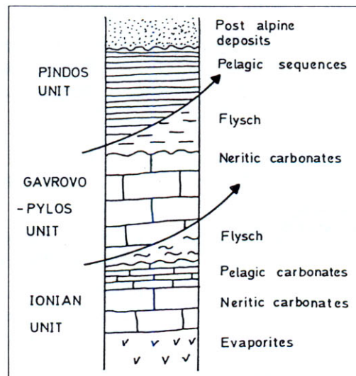
Figure 2 - Les unités géotectoniques du Péloponnèse occidentale - The geotectonic units in western Peloponnese.
